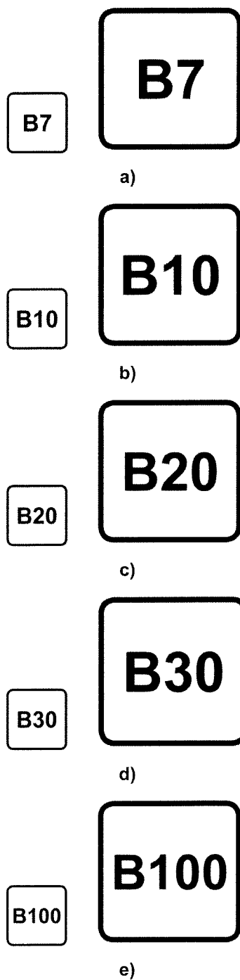
Фигура А.2 – Пример за идентификатори за смеси на FAME
